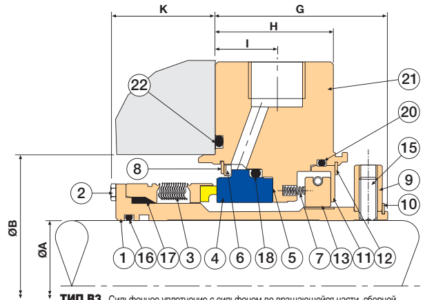
ТИП В3 - Сильфонное уплотнение с сильфоном во вращающейся части, сборной подвижной дроссельной втулкой и механически фиксированным стационарным кольцом пары трения
